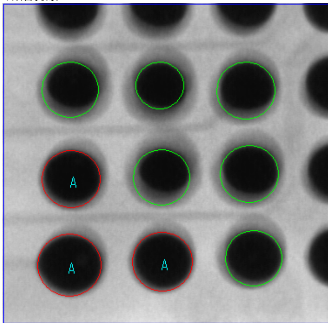
管電圧62kV 倍率40倍 A部ボール浮き上がり
