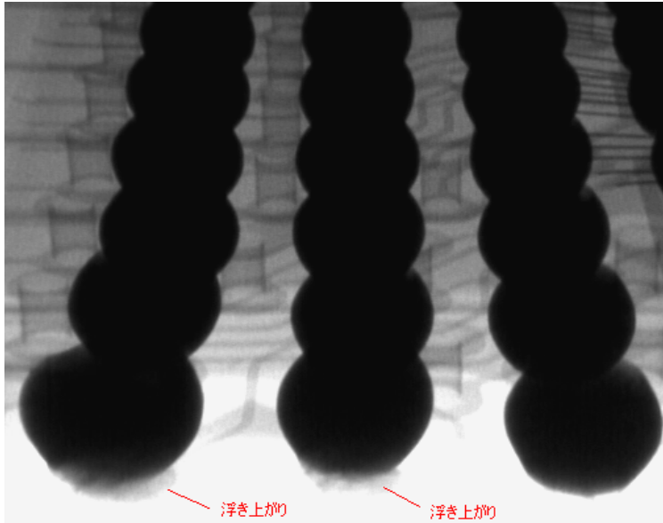
管電圧57kV 倍率75倍
